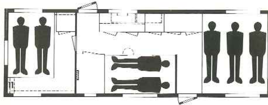
UITVOERING 760 TA/a
