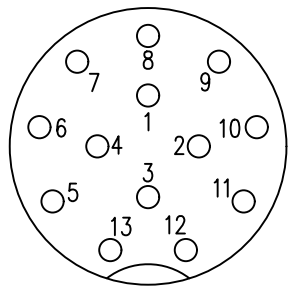
Achterzijde/Rückseite
